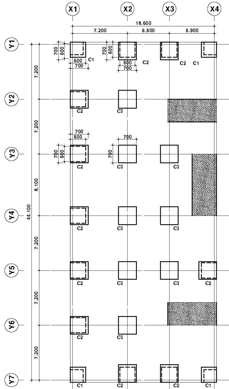
주심도 축척: 1/200, 1/60
