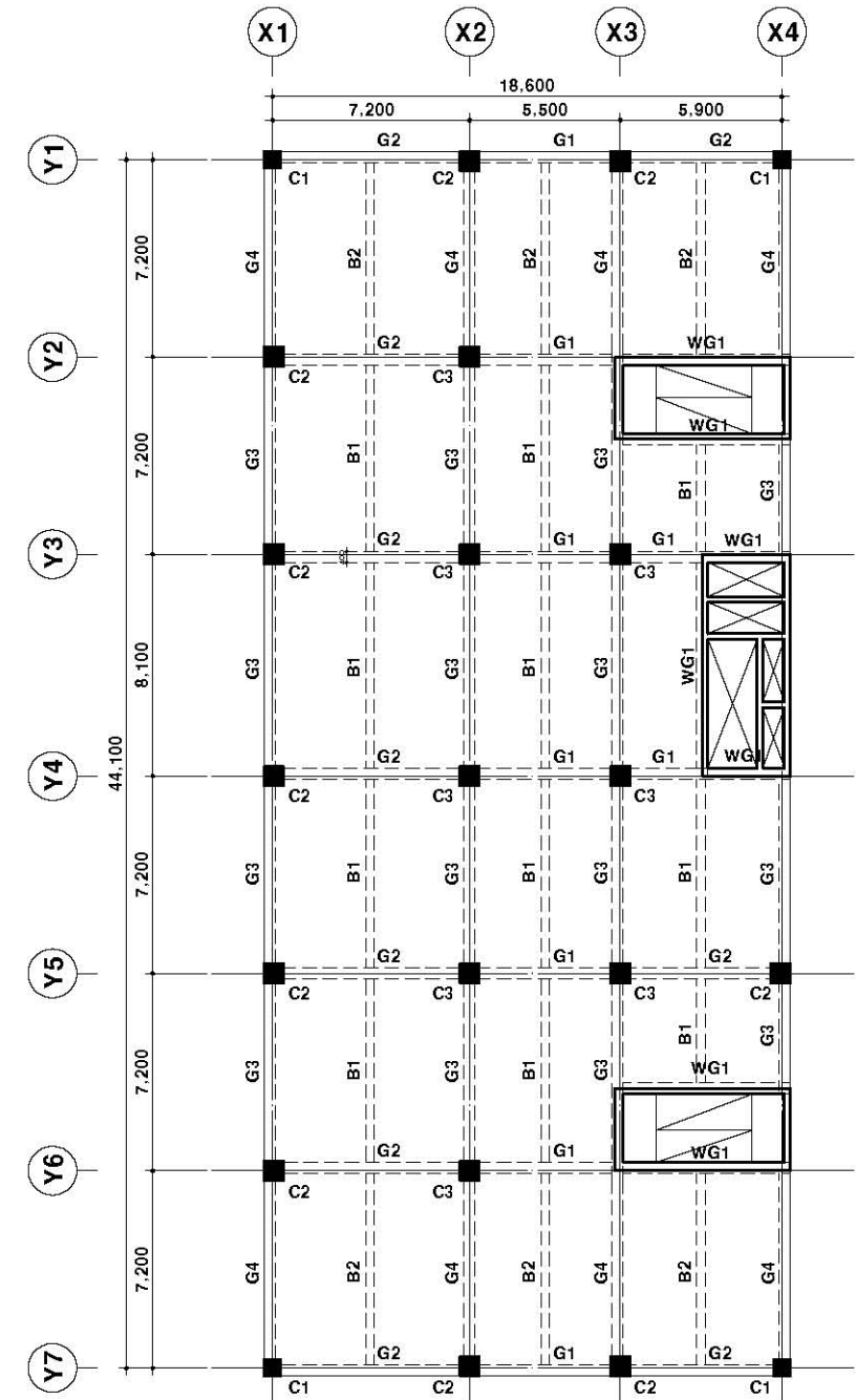
지상 4층 구조평면도 축척: 1/200
