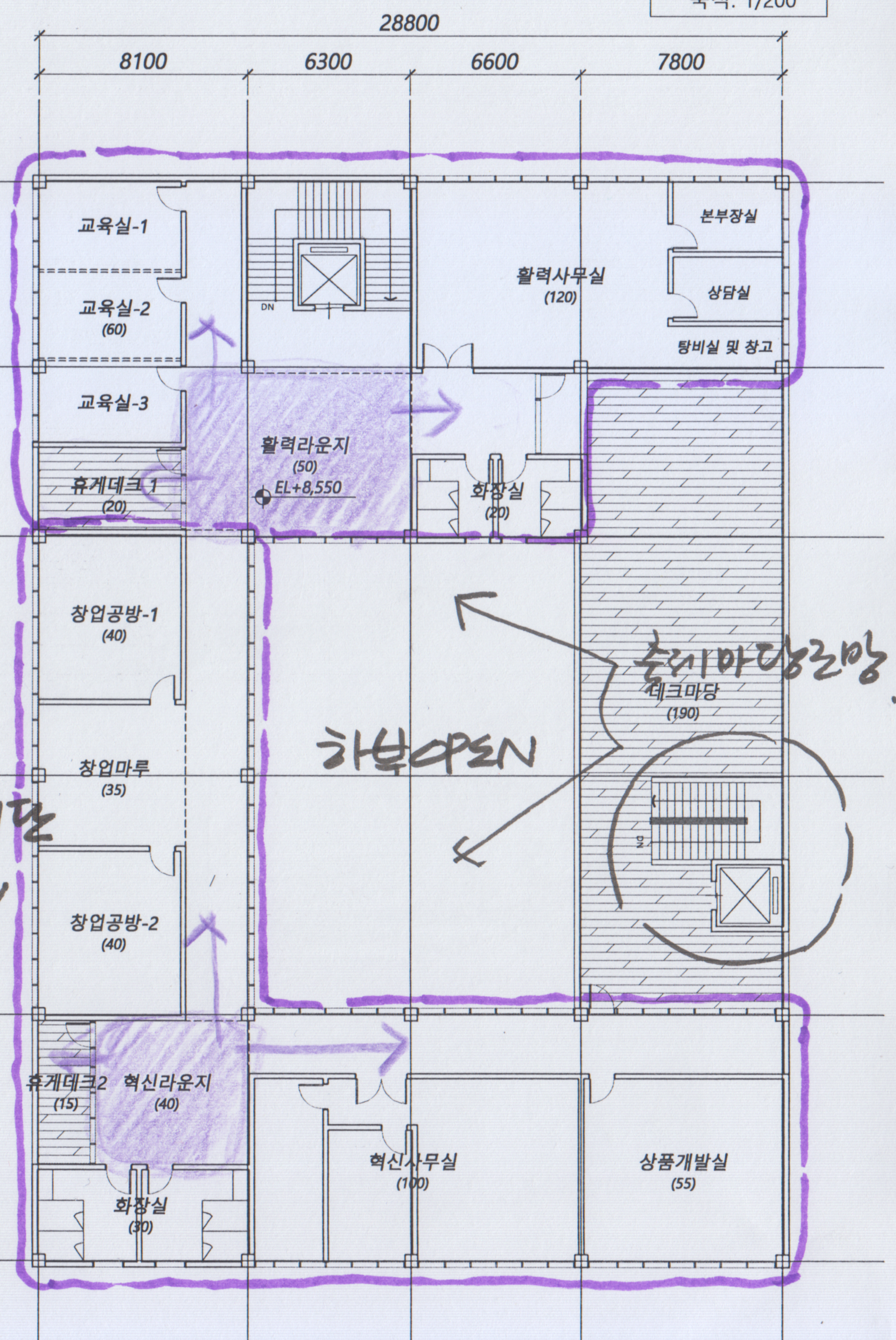
지상 2층 평면도 축척: 1/200
