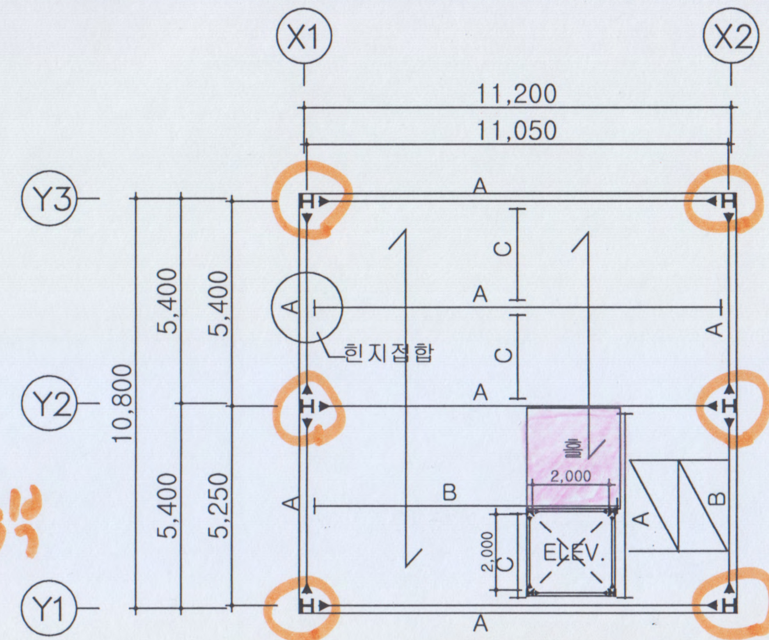
지상 6층 구조평면도 축척: 1/150
