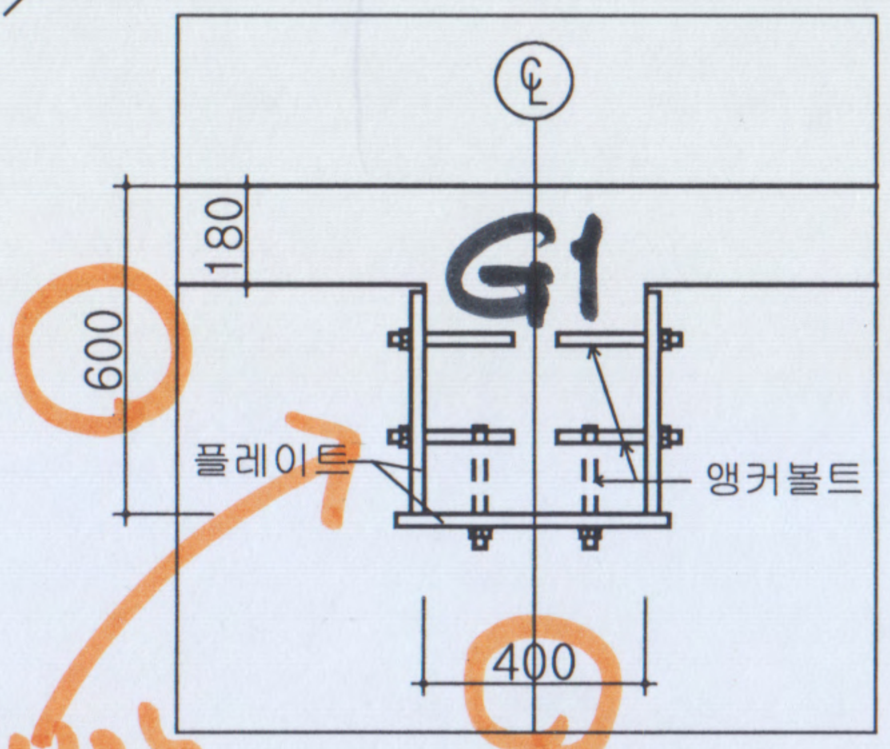
구조보강 단면상세도 축척: 1/20
