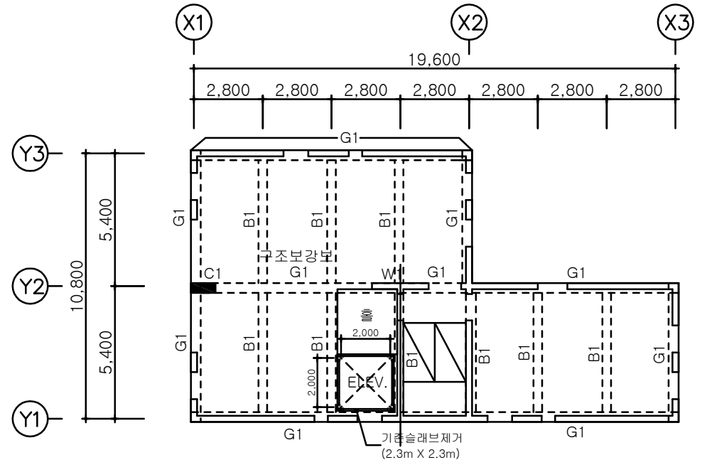
지상 3층 구조평면도 축척: 1/150
