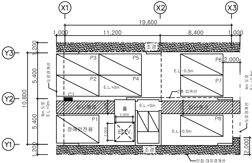
지상 1층 평면도 축척: 1/150
