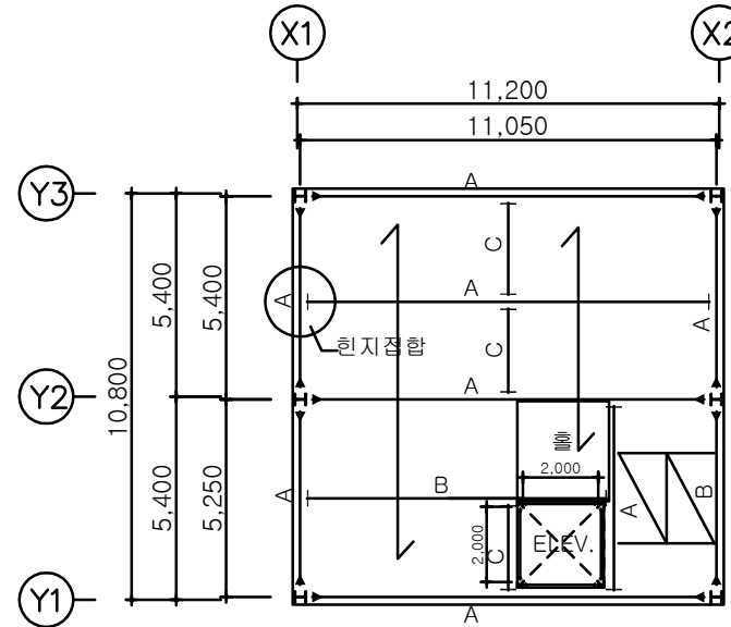
지상 6층 구조평면도 축척: 1/150
