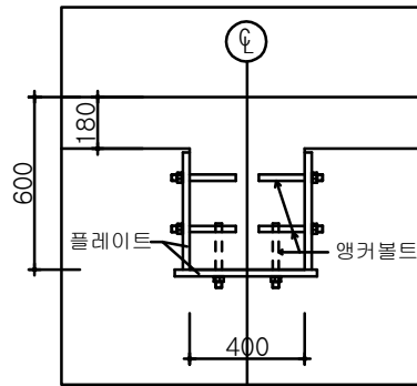
구조보강 단면상세도 축척: 1/20
