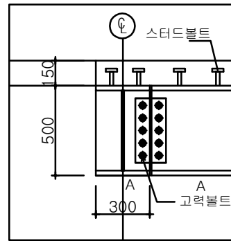
접합부 단면상세도 축척: 1/20
