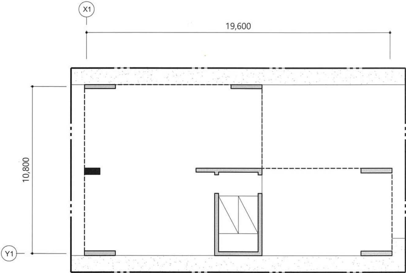
지상 1층 평면도 축척: 1/150
