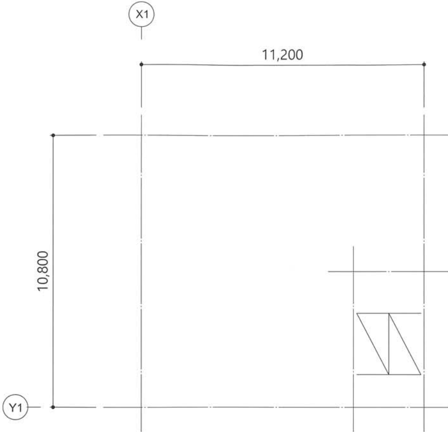
지상 6층 구조평면도 축척: 1/150
