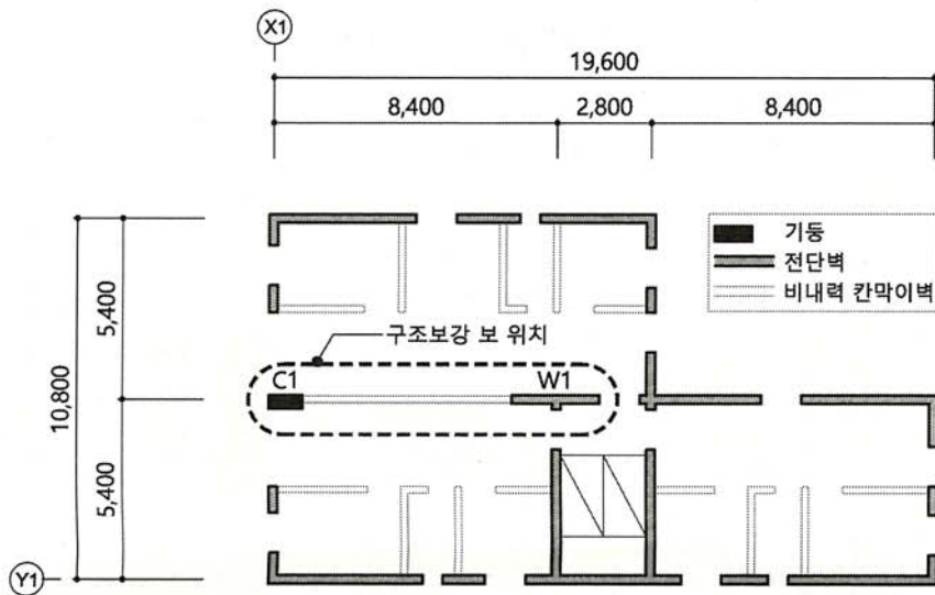
지상 2층~4층 평면도
