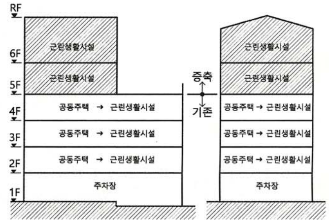
A-A' 단면 개념도
