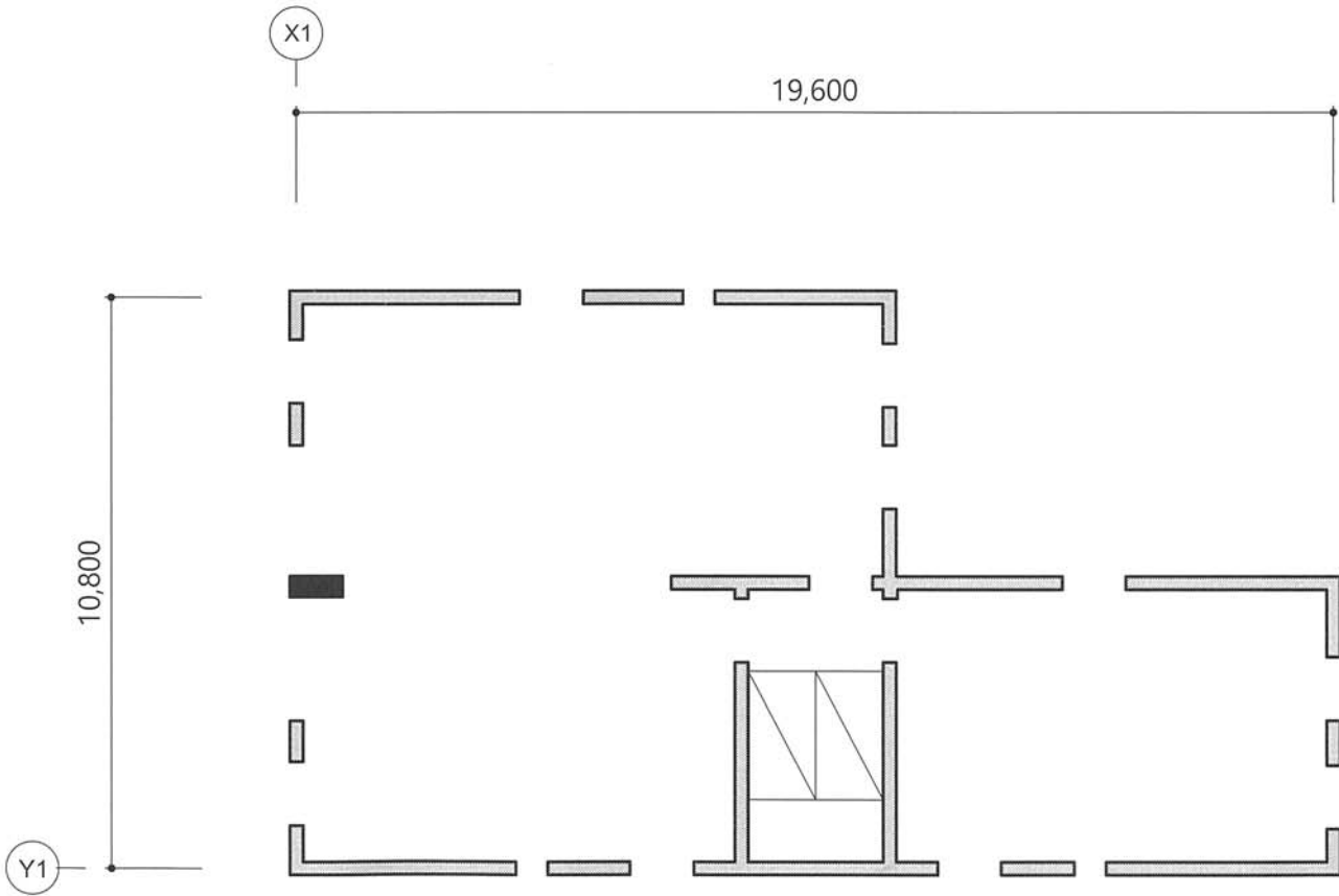
지상 3층 구조평면도 축척: 1/150
