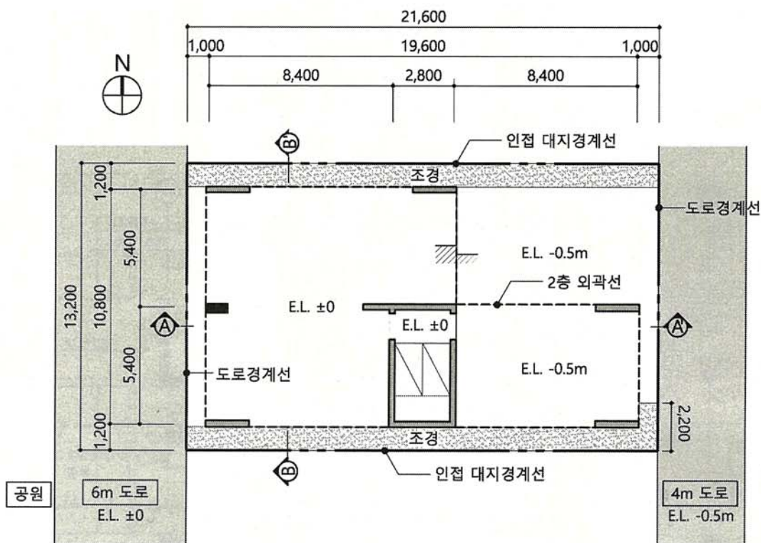
지상 1층 평면도
