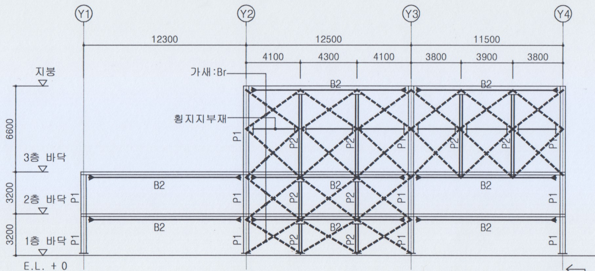
A-A' 구조 입면도 축척: 1/200
