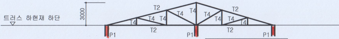
트러스 입면도 축척: 1/200
