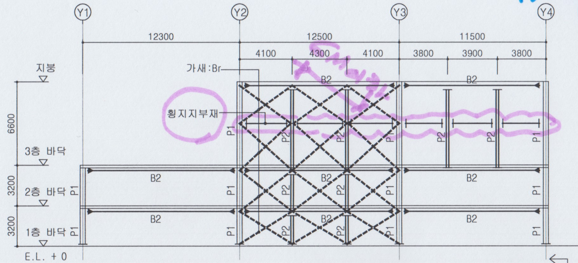
A-A' 구조 입면도
