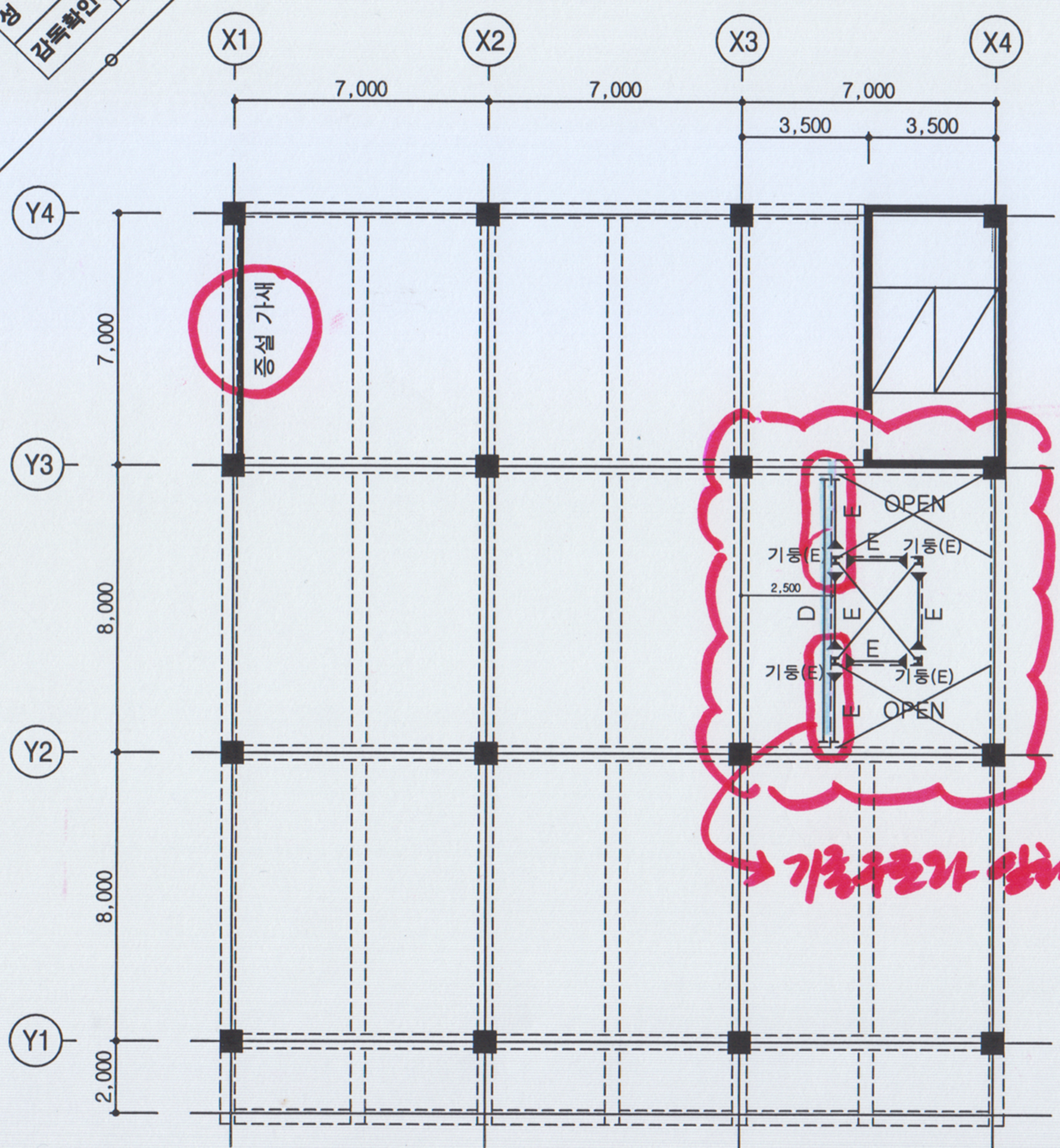
지상 4층 구조평면도 축척: 1/150
