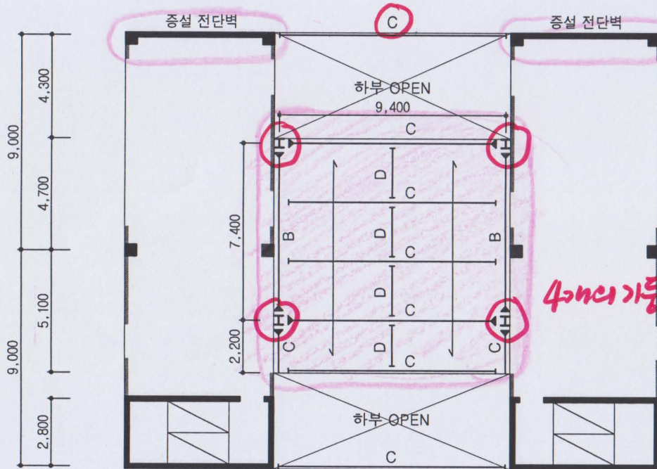
2층 구조평면도 축척: 1/150
