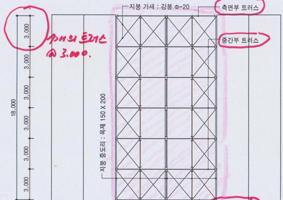
지붕 구조평면도 축척: 1/150
