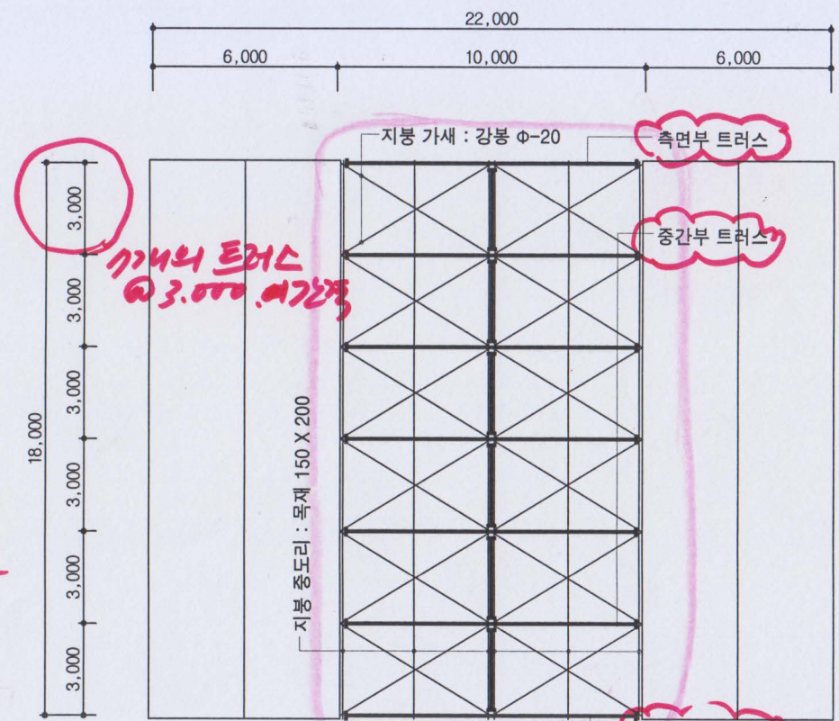
지붕 구조평면도 축척: 1/150
