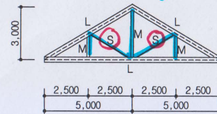
중간부 트러스 입면도 축척: 1/150
