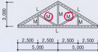
측면부 트러스 입면도 축척: 1/150
