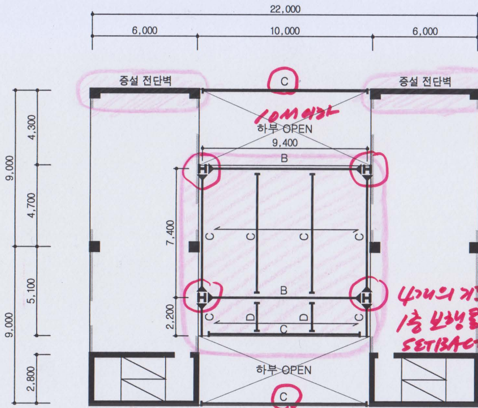
2층 구조평면도 축척: 1/150
