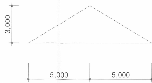
중간부 트러스 입면도 축척 : 1/150
