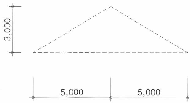
측면부 트러스 입면도 축척 : 1/150
