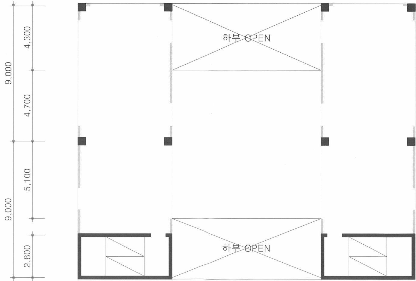
2층 구조평면도 축척 : 1/150
