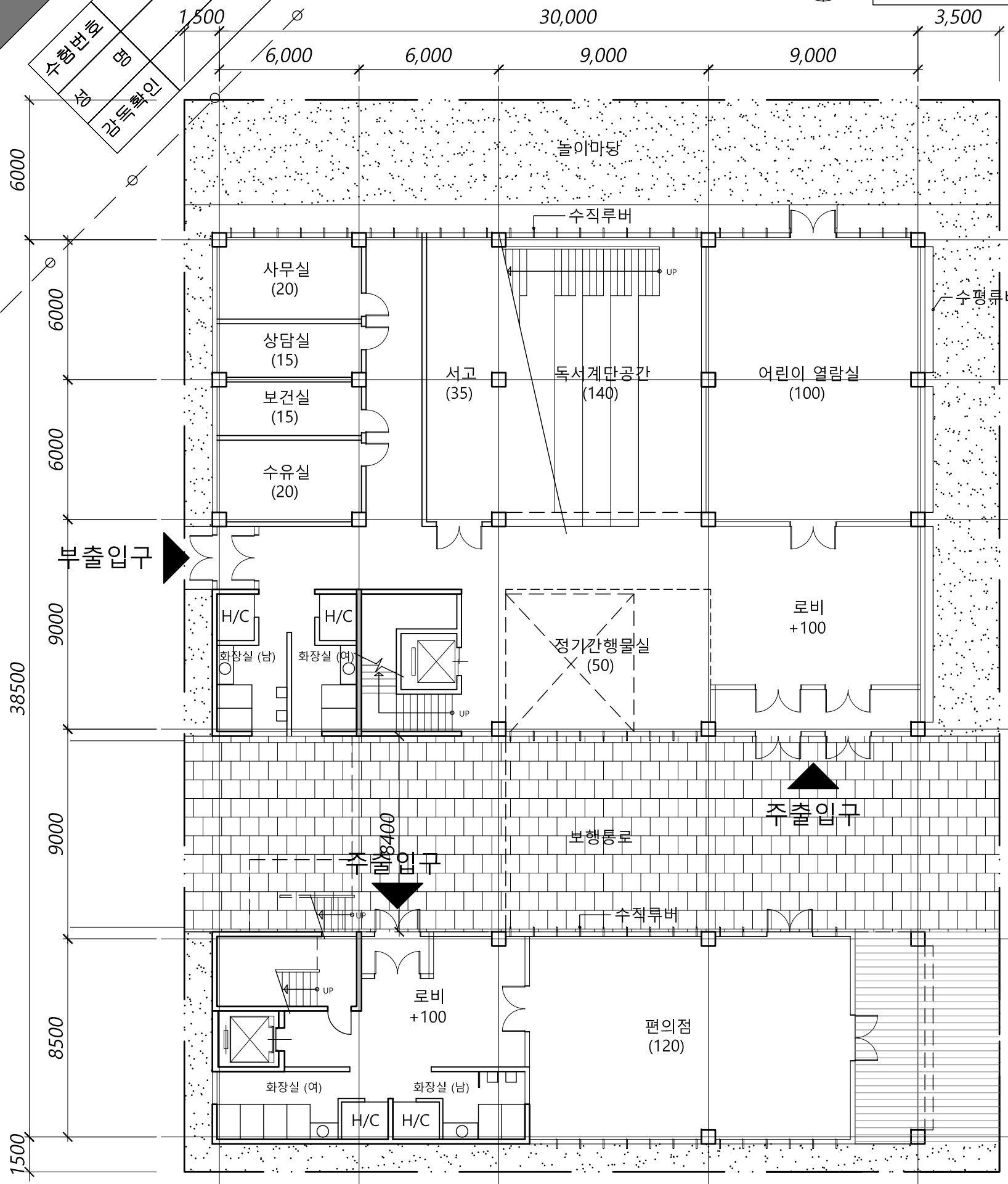
1층 평면도 축척 : 1/200
