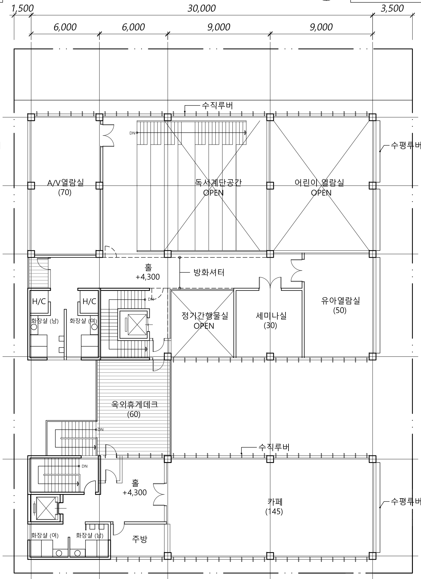
2층 평면도 축척 : 1/200
