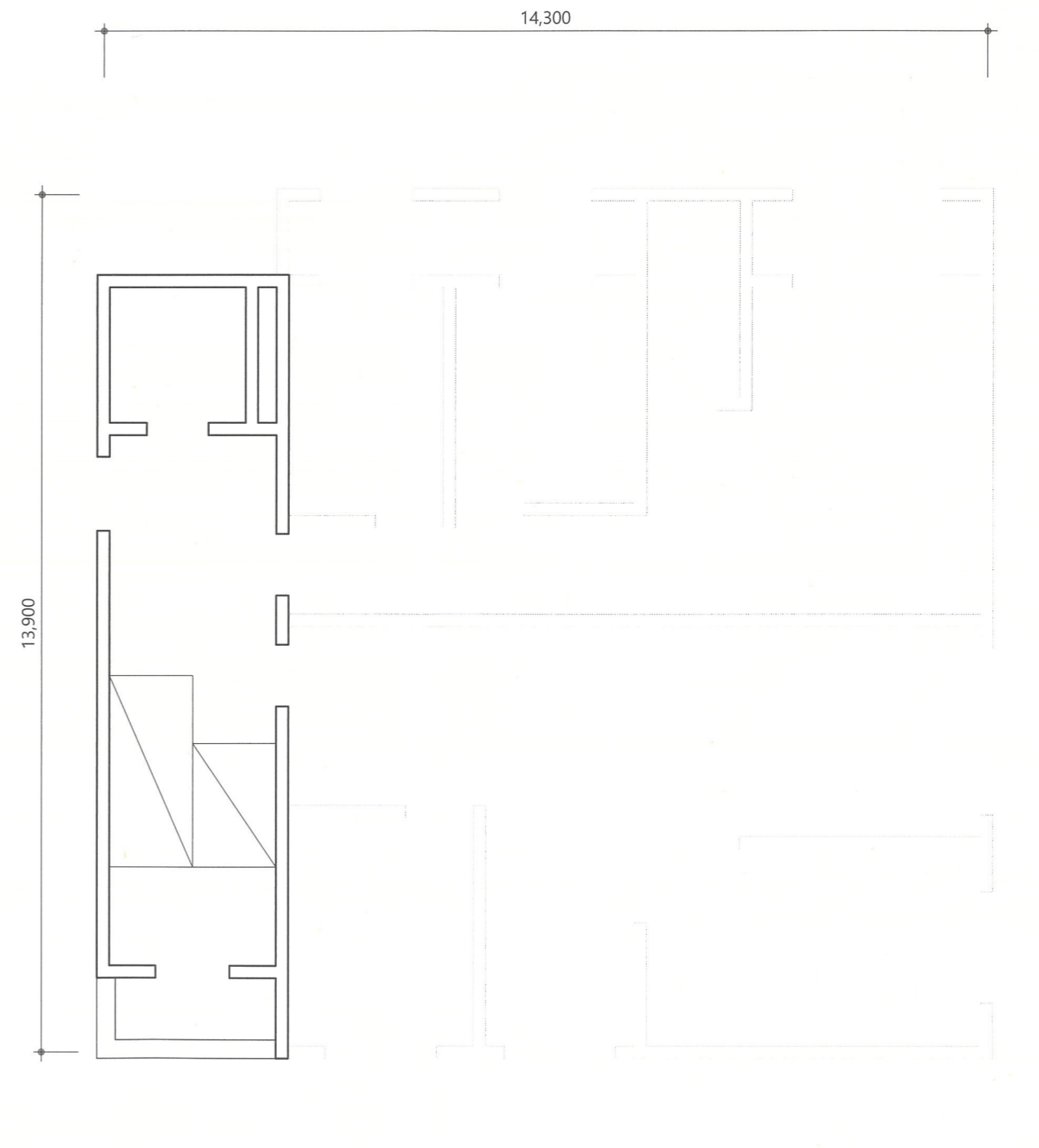
3층 구조평면도 축척 : 1/100
