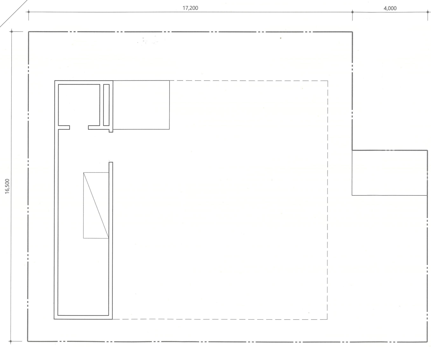
1층 구조평면도 축척 : 1/100
