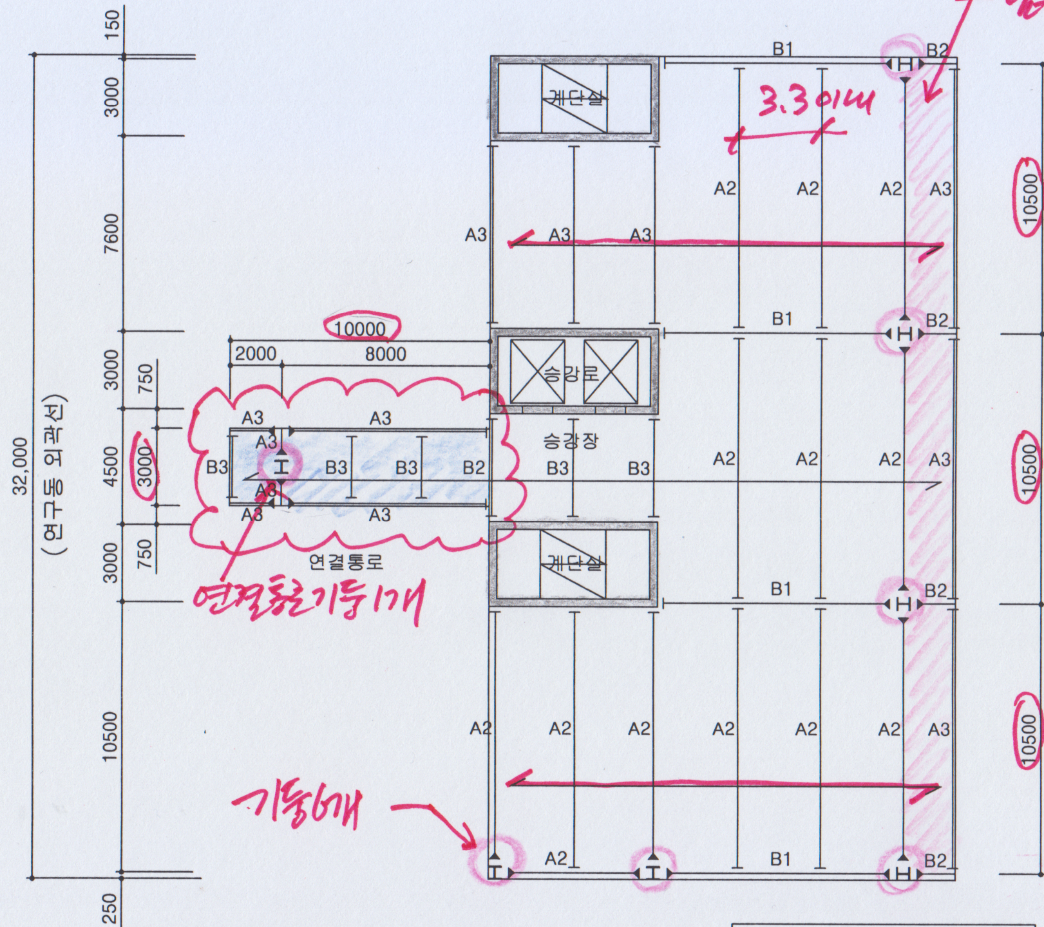
지상 2층 구조 평면도 축척: 1/200
