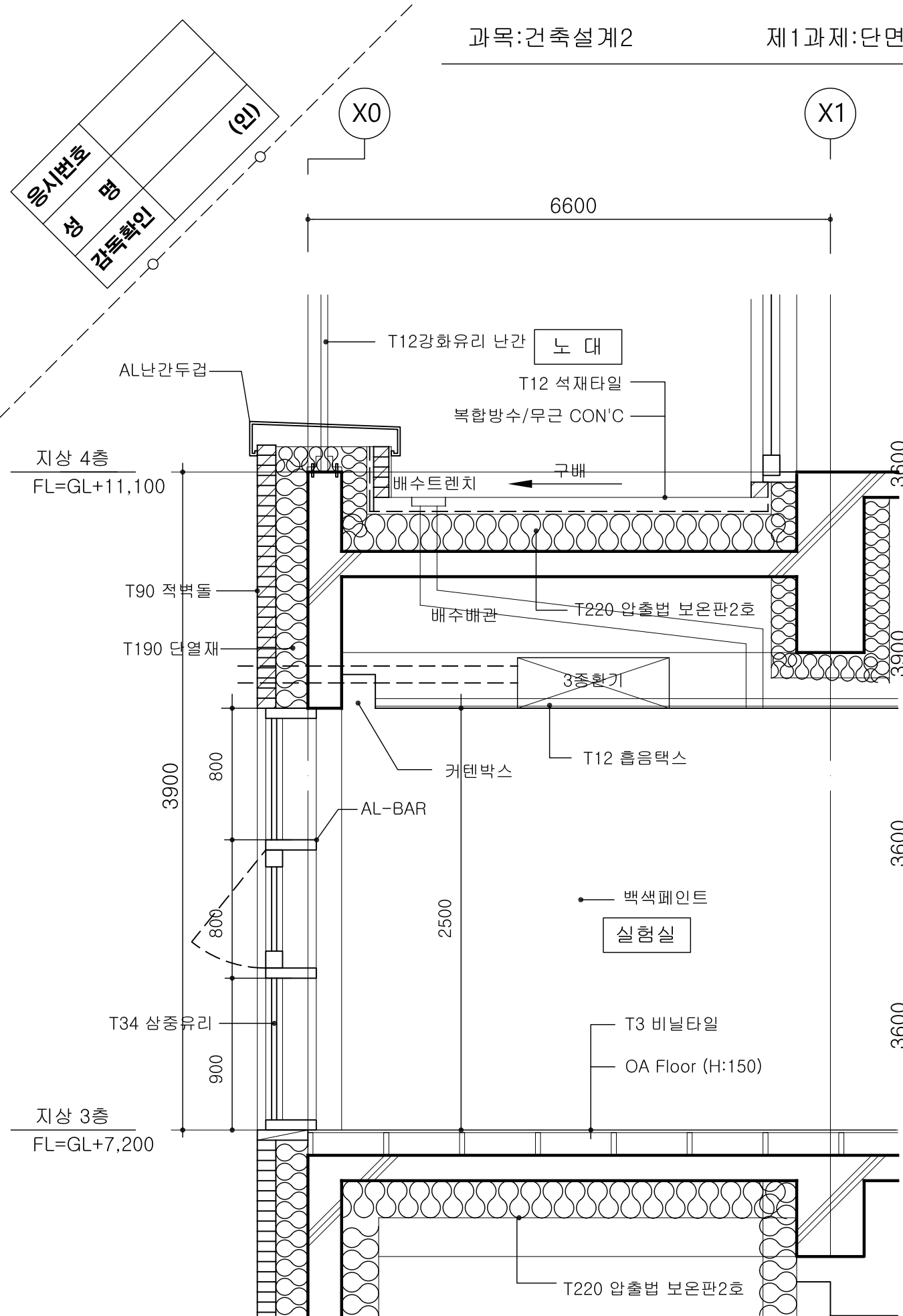
B부분 단면상세도 축척:1/30
