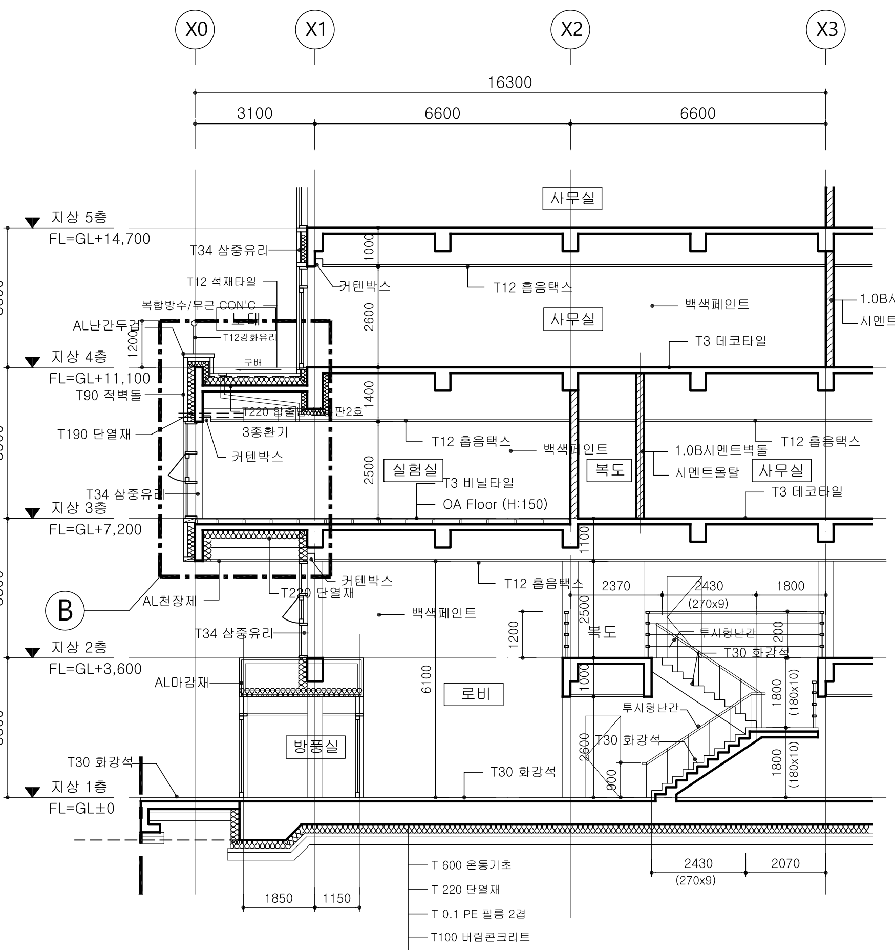
A-A' 부분단면도 축척:1/100
