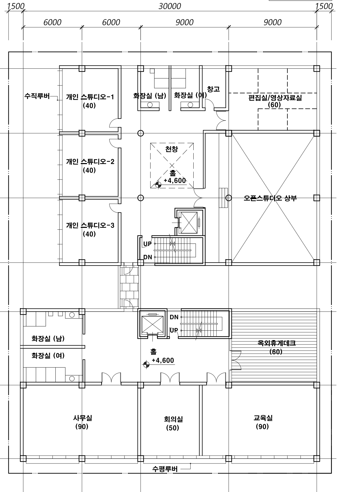
2층 평면도
