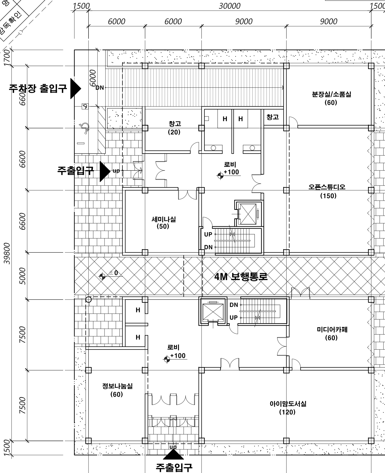
1층 평면도
