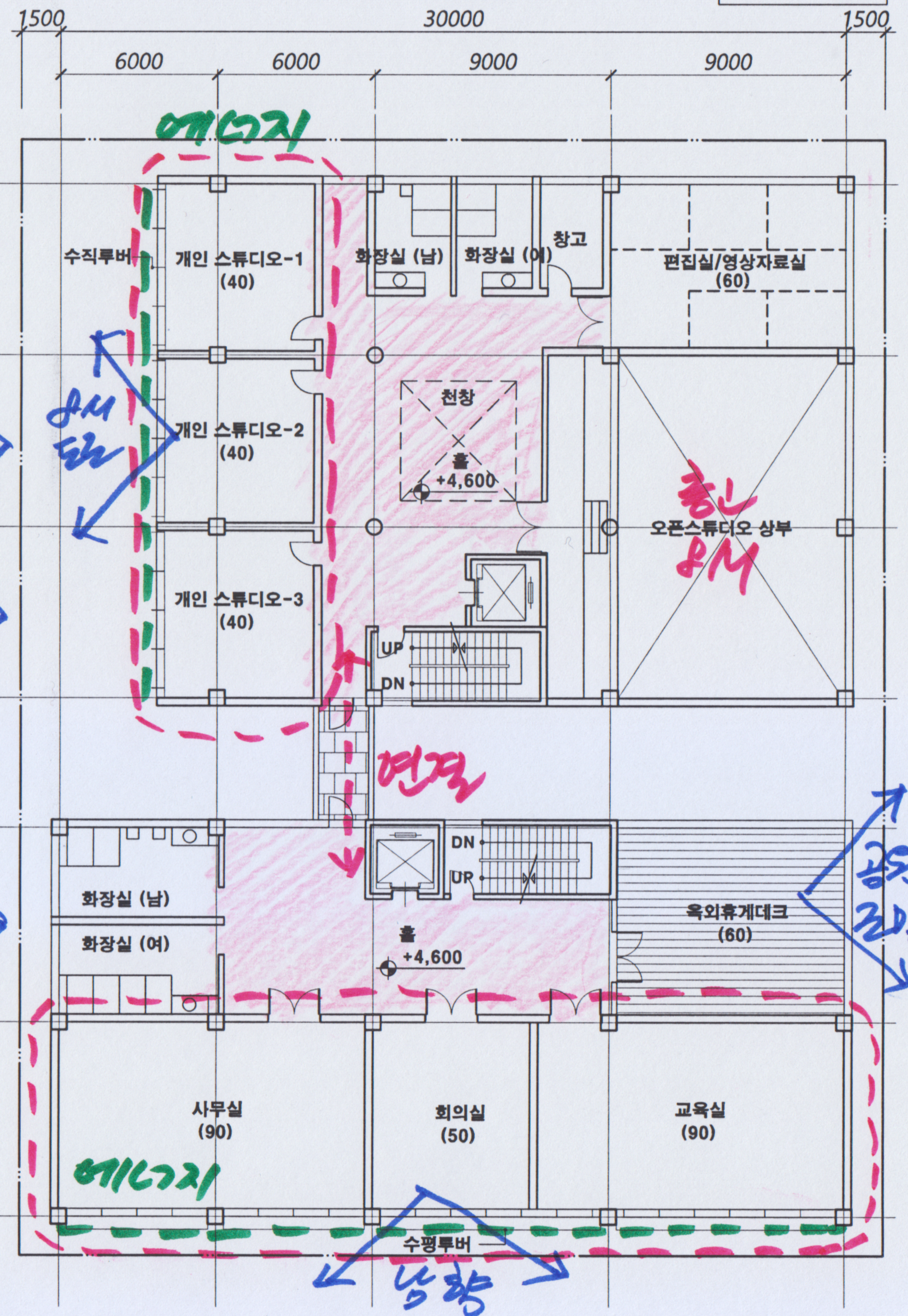
2층 평면도 축척: 1/200
