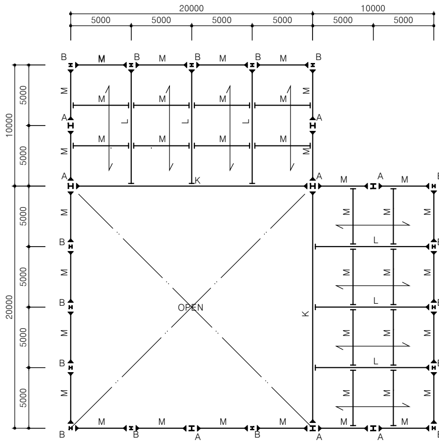
2층 구조평면도 축척: 1 / 200
