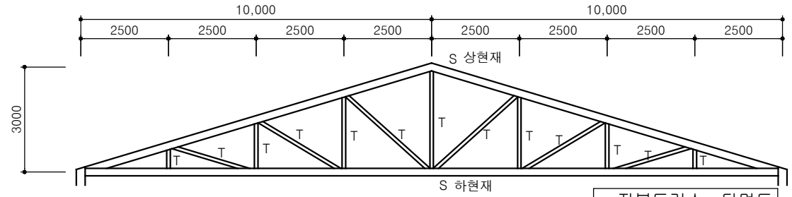
지붕트러스 단면도 축척: 1 / 100
