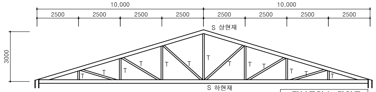
지붕트리스 단면도 축척: 1/100
