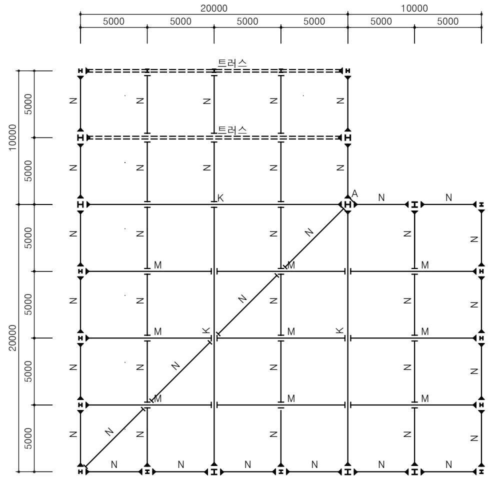
지붕 구조평면도 축척: 1/200
