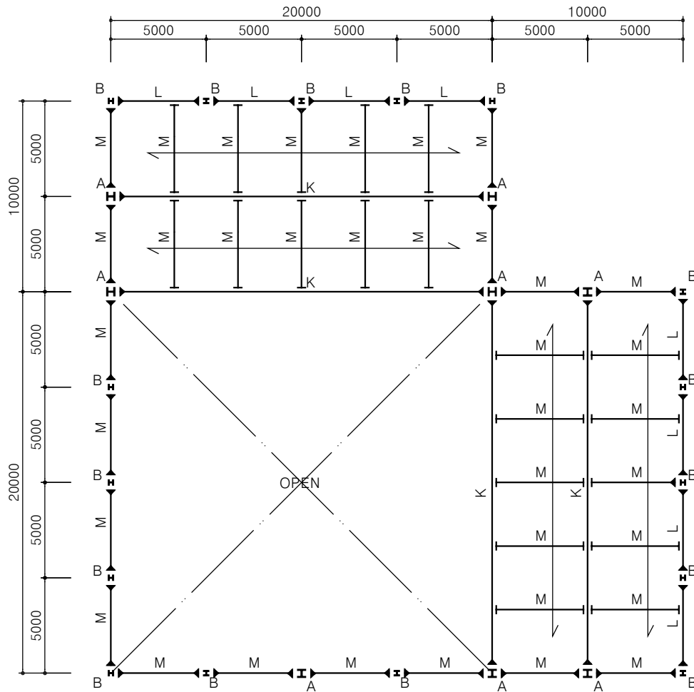
2층 구조평면도 축척: 1/200
