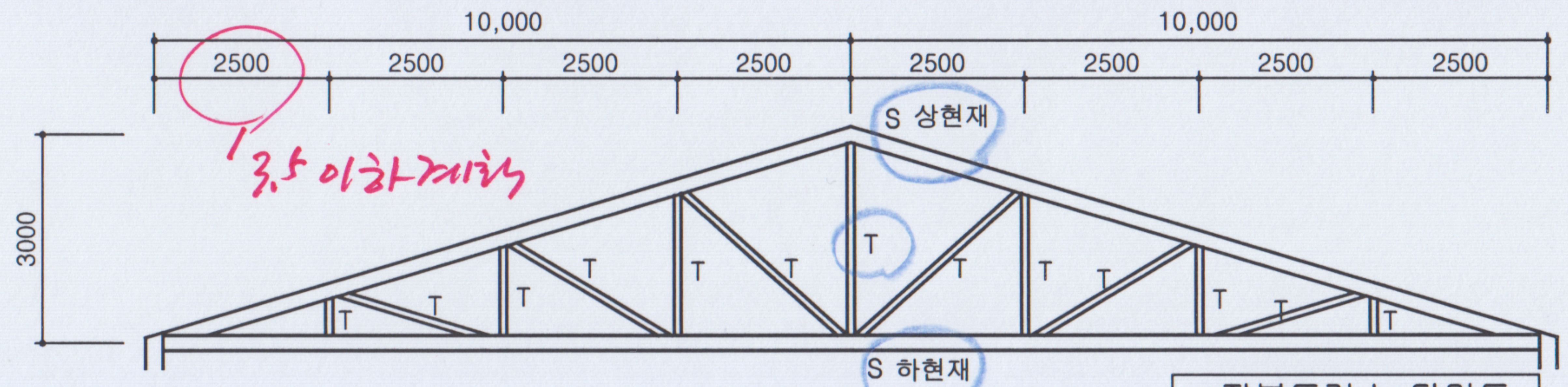
지붕트러스 단면도 축척: 1/100
