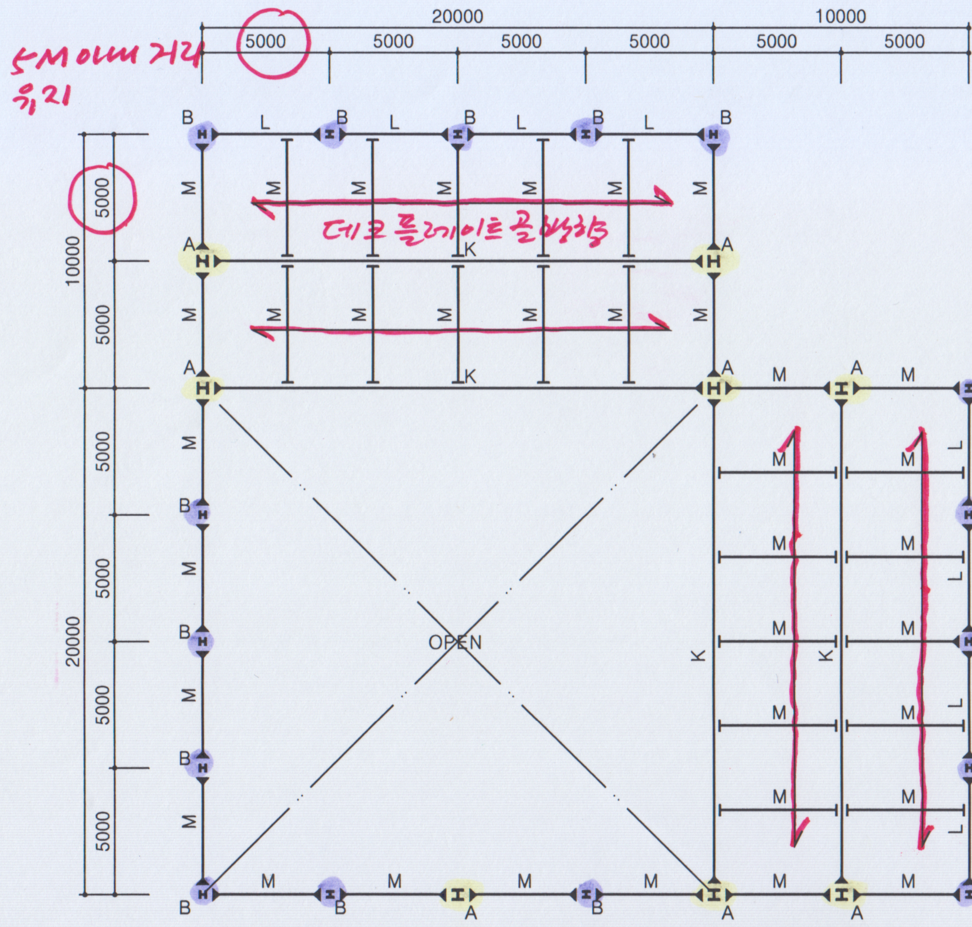
2층 구조평면도 축척: 1/200
