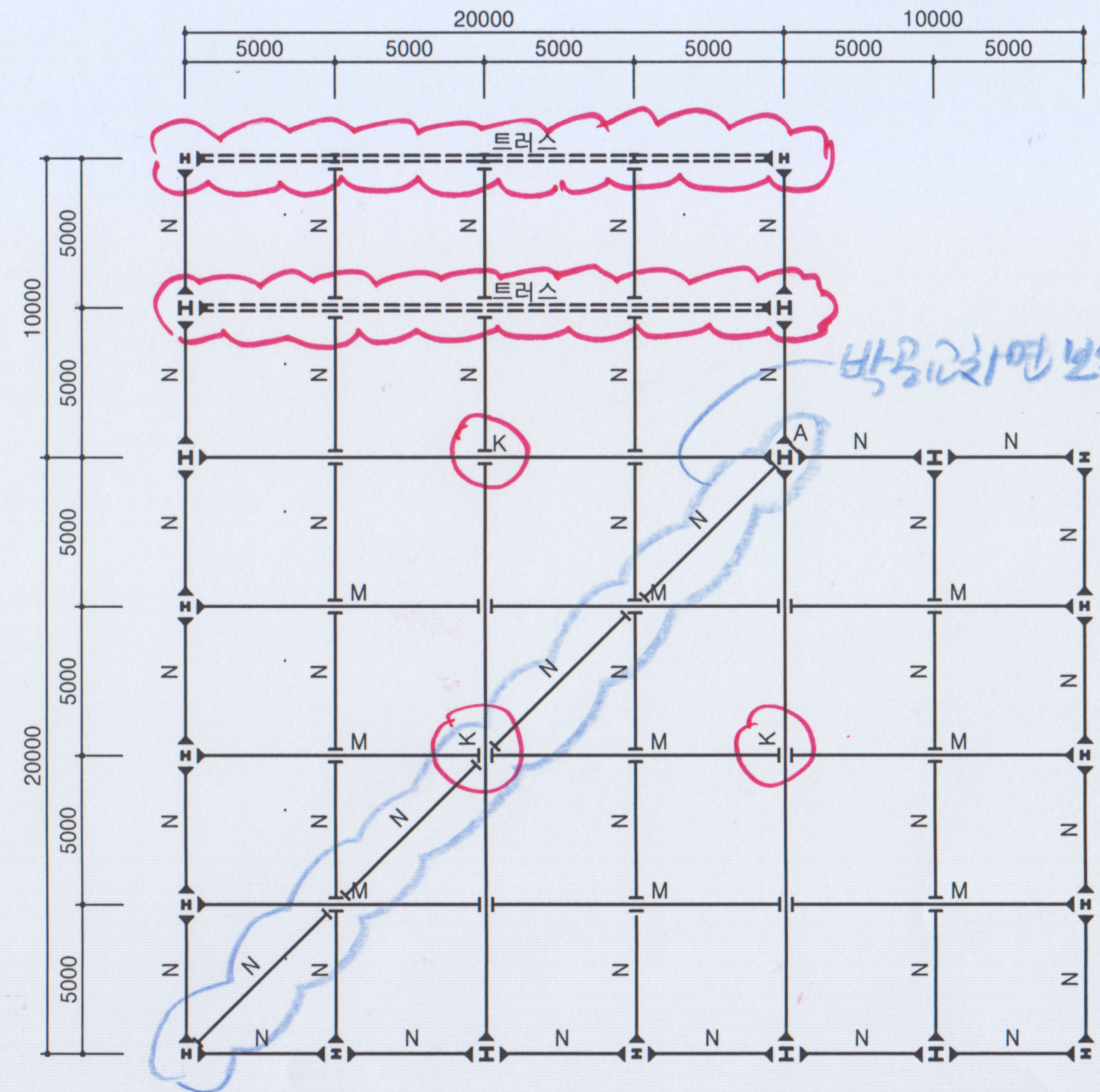
지붕 구조평면도 축척: 1/200
