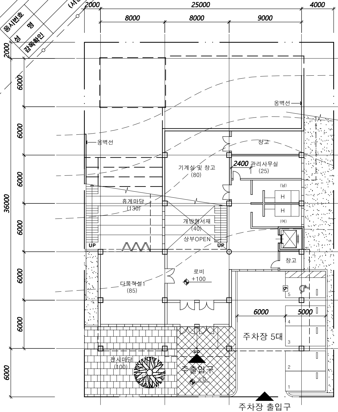
1층 평면도 축척: 1/200
