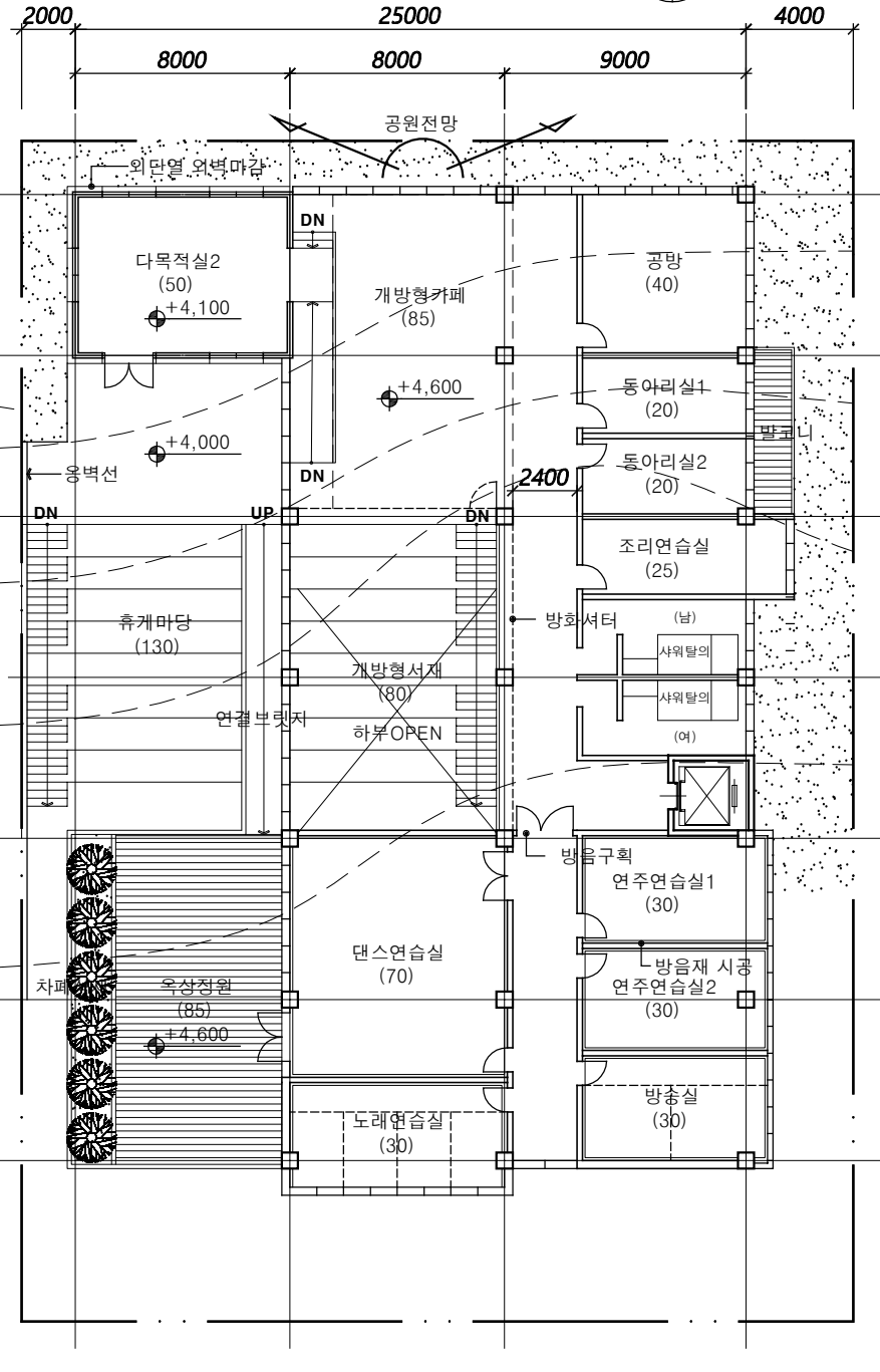
2층 평면도 축척: 1/200
