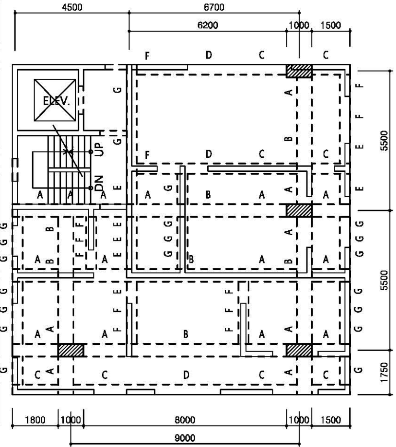
2층 구조 평면도 축척:1/100
