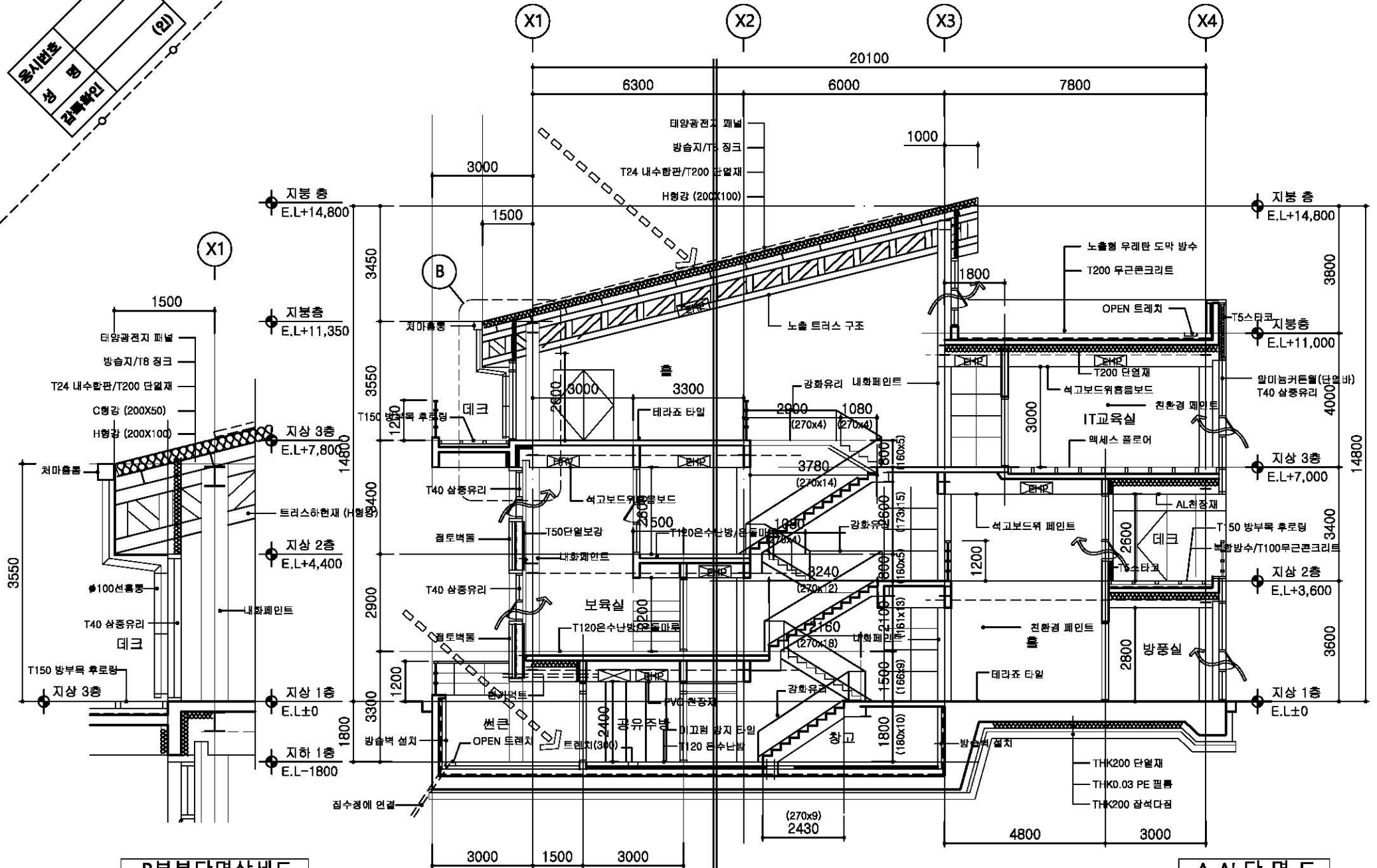
B부분단면상세도 축척:1/50
