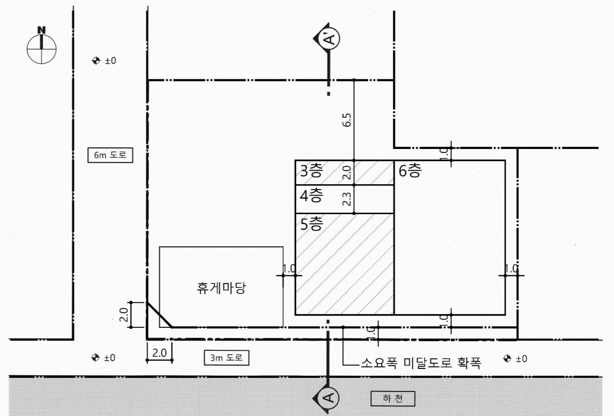
배치도 축척: 1/300
