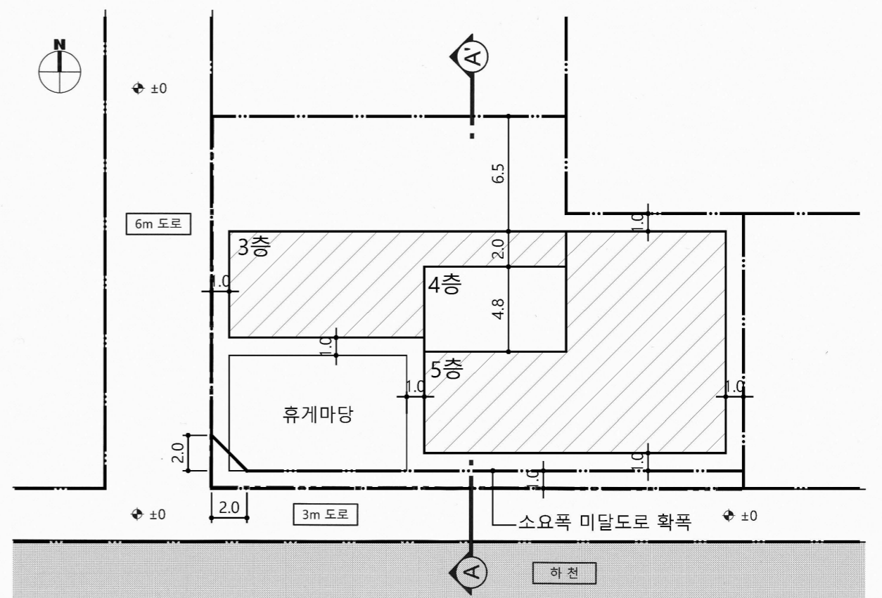
배치도 축척: 1/300
