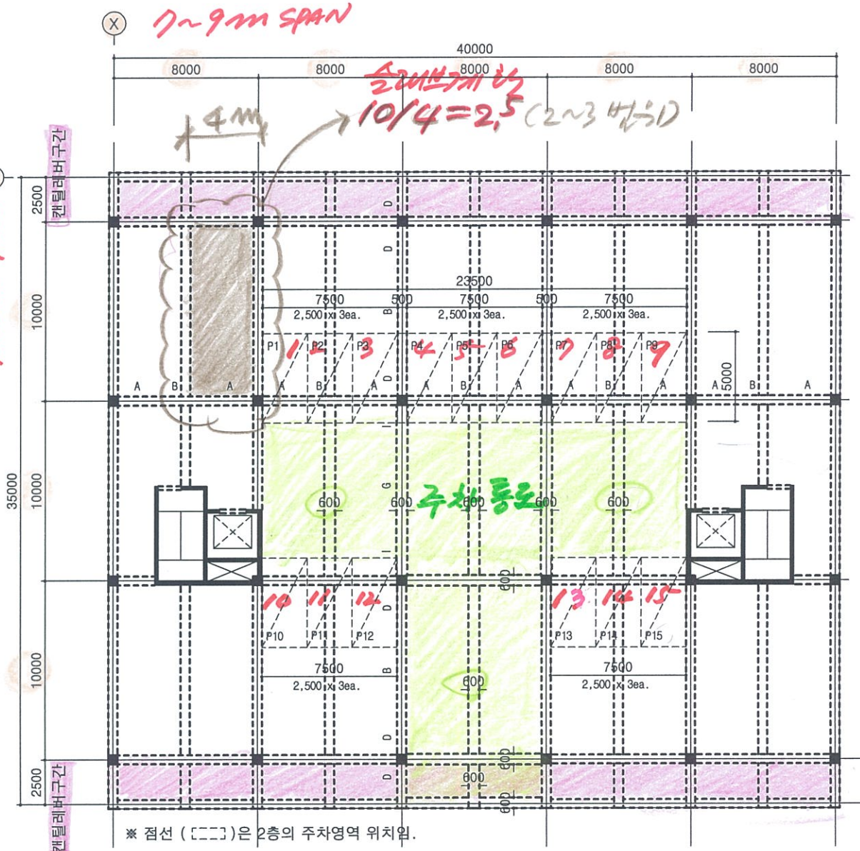
3층 구조평면도 축척: 1/200
