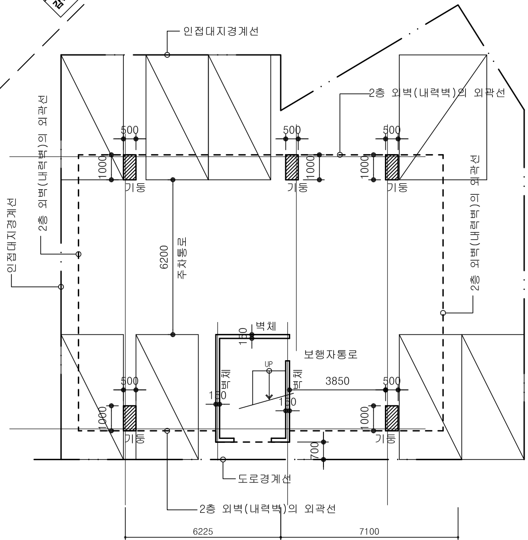
1층 평면도 축척: 1/100
