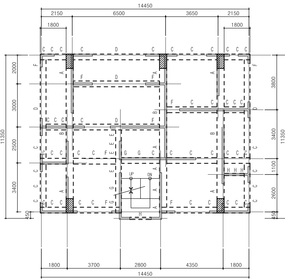
2층 구조 평면도 축척: 1/100
