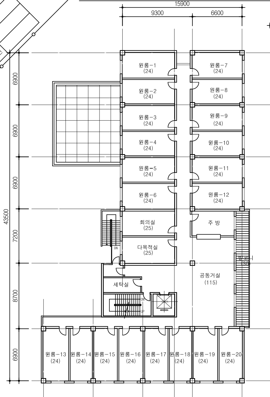
2층 평면도
