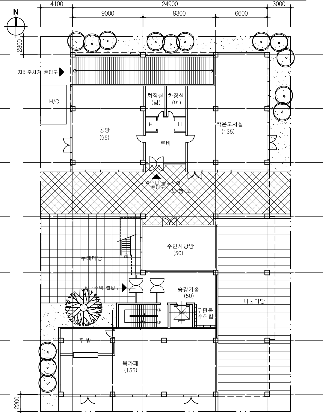
1층 평면도
