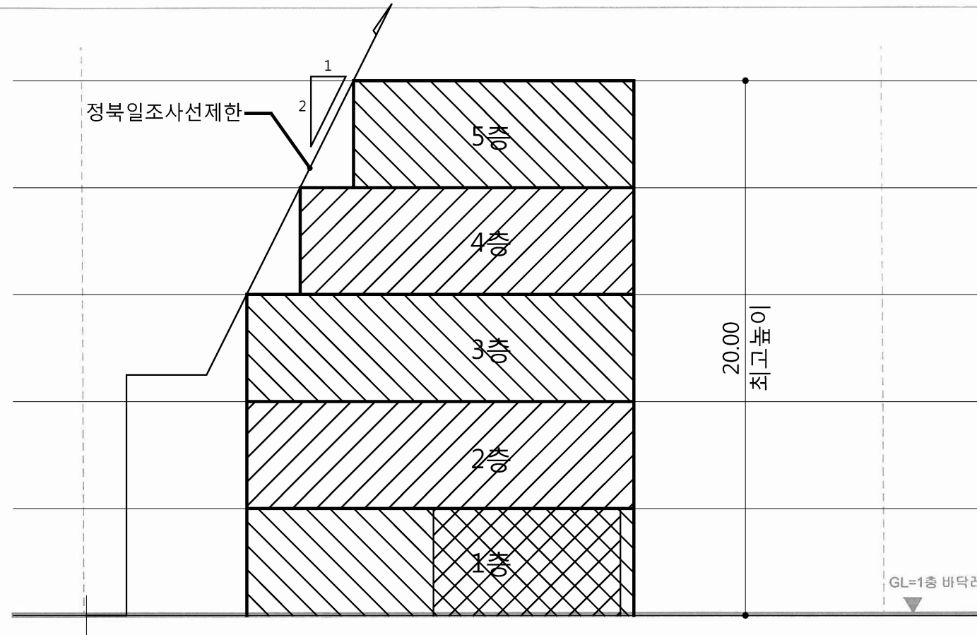
X-X' 단면도 축척:1/200
