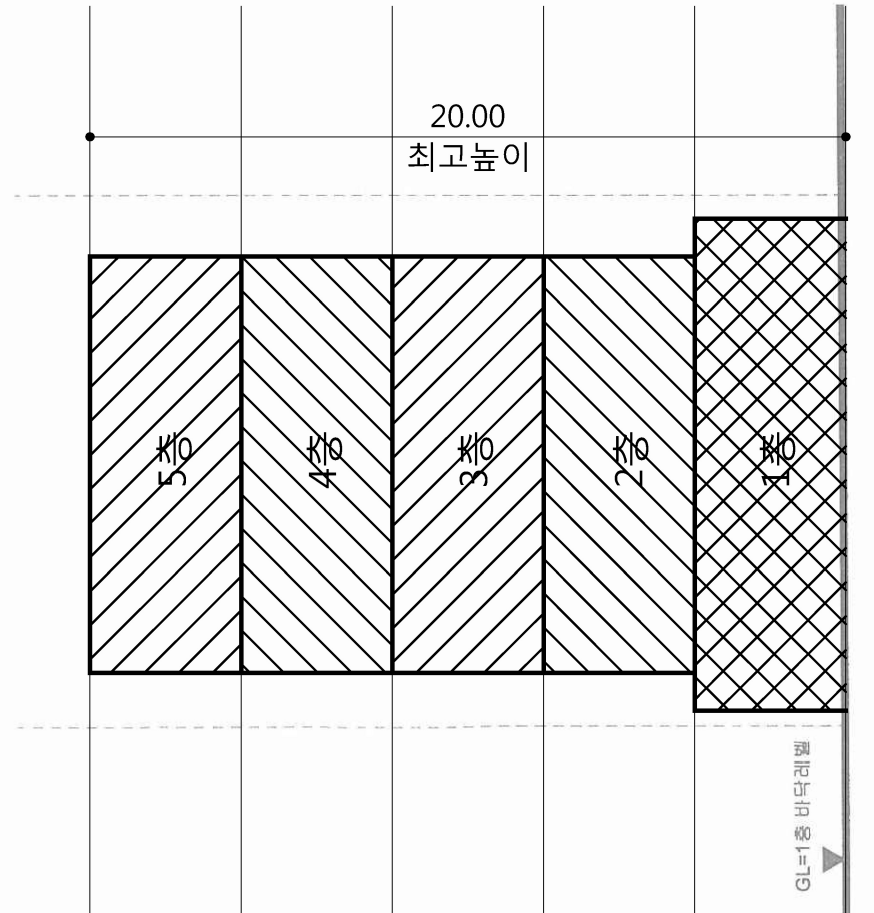
X-X' 단면도 축척:1/200
