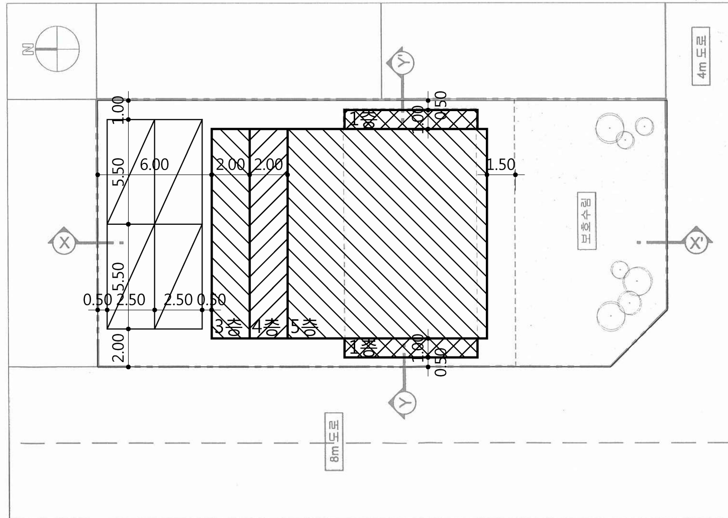
배치도 축척:1/200
