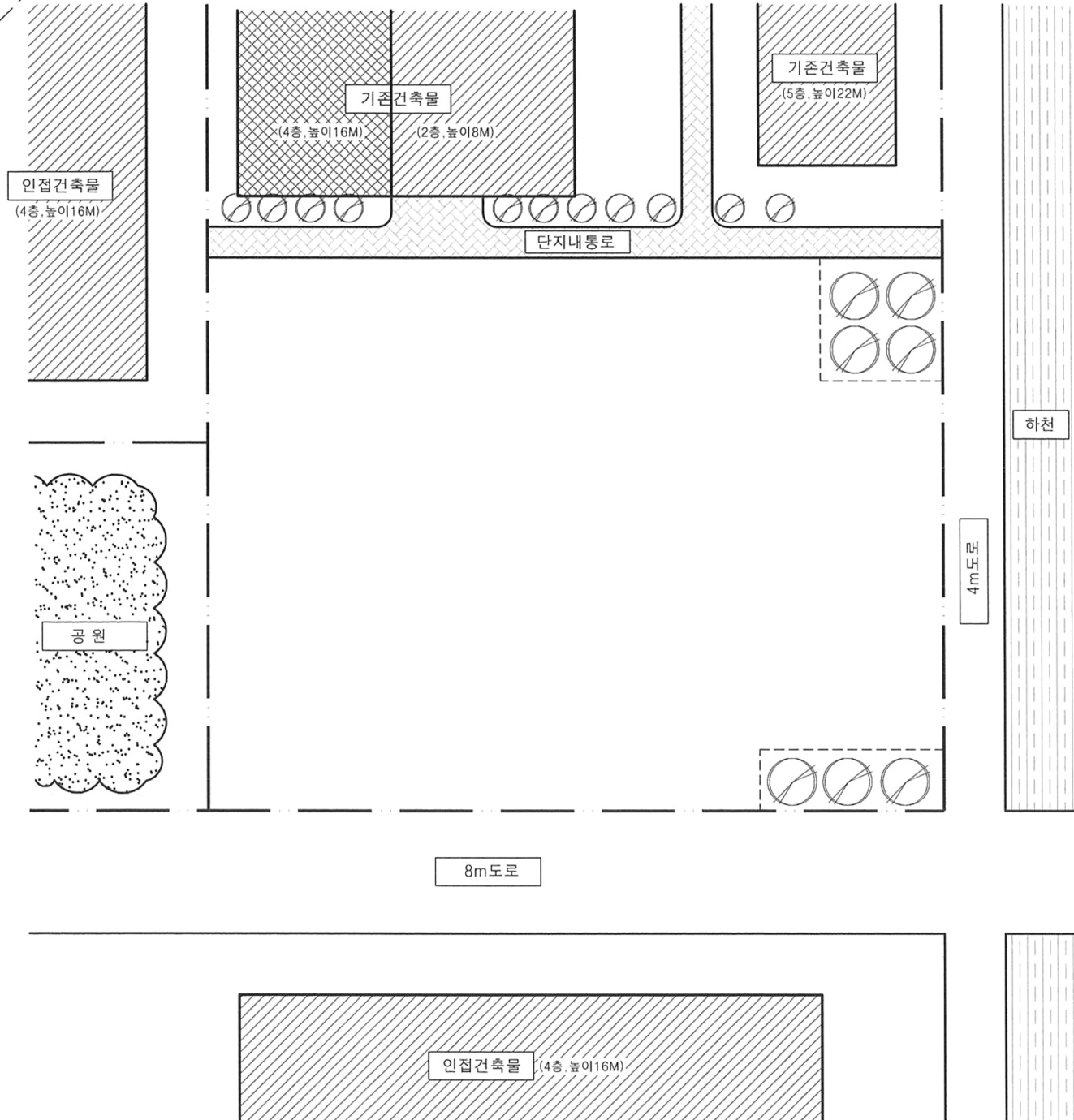
배치도 축척 : 1/400
