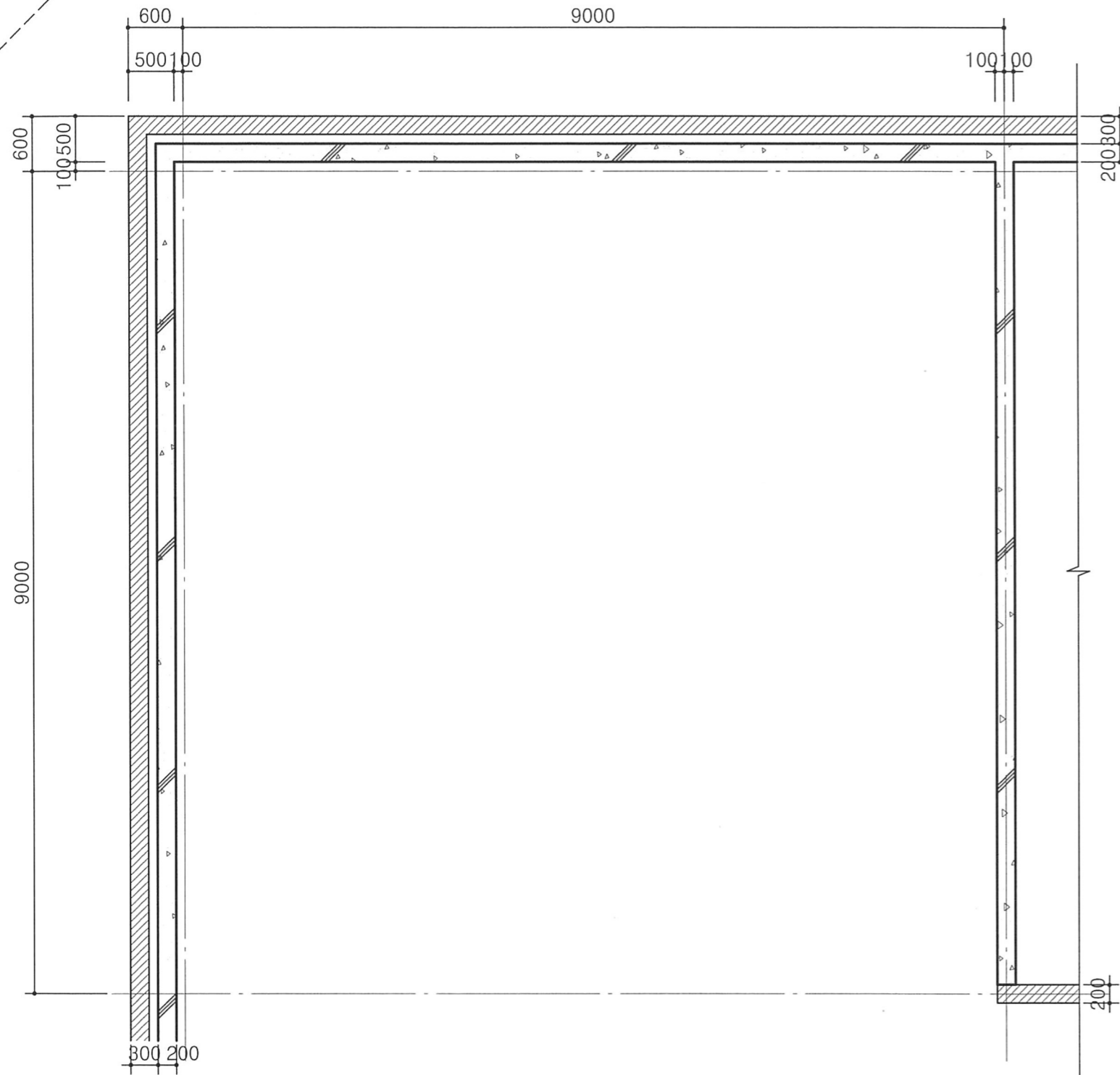
5층계단평면도 축척 : 1/60
